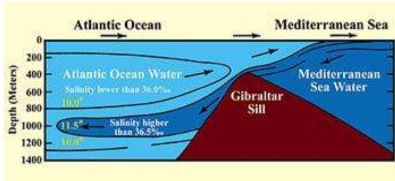
Figura 1. Marea Mediterană atunci când intră în Atlantic prin strâmtoarea Gibraltar cu apa ei caldă, sărată și mai puțin densă din cauza barierei care face diferența dintre ele. Temperatura este în Celsius. (Marine Geology, Keunen, p.43)
